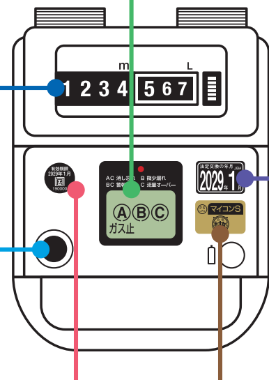
マイコンメーターSの例
