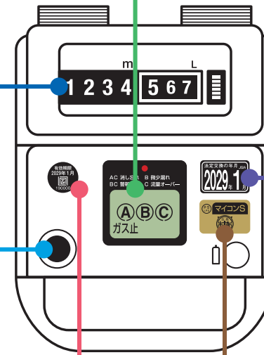
マイコンメーターSの例
